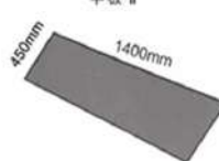
Flat Sheet II 平板 II
