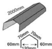
Angle Ridge Cap I 角型脊瓦 I
