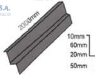
Wall Side Flashing 泛水板
