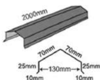
Angle Ridge Cap 角型脊瓦 II
