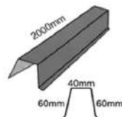
Square Ridge Cap 方型脊瓦
